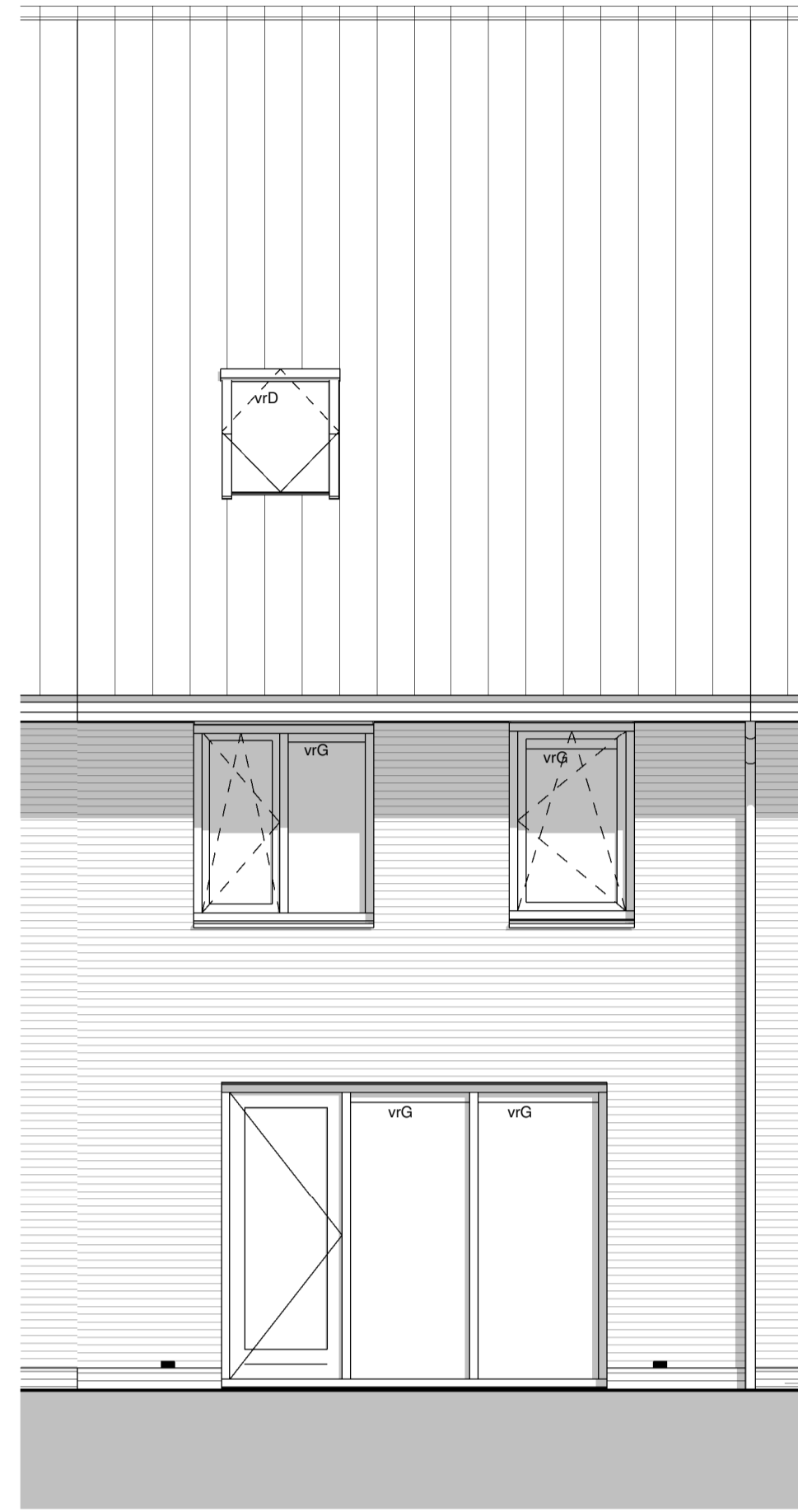
Achtergevel
