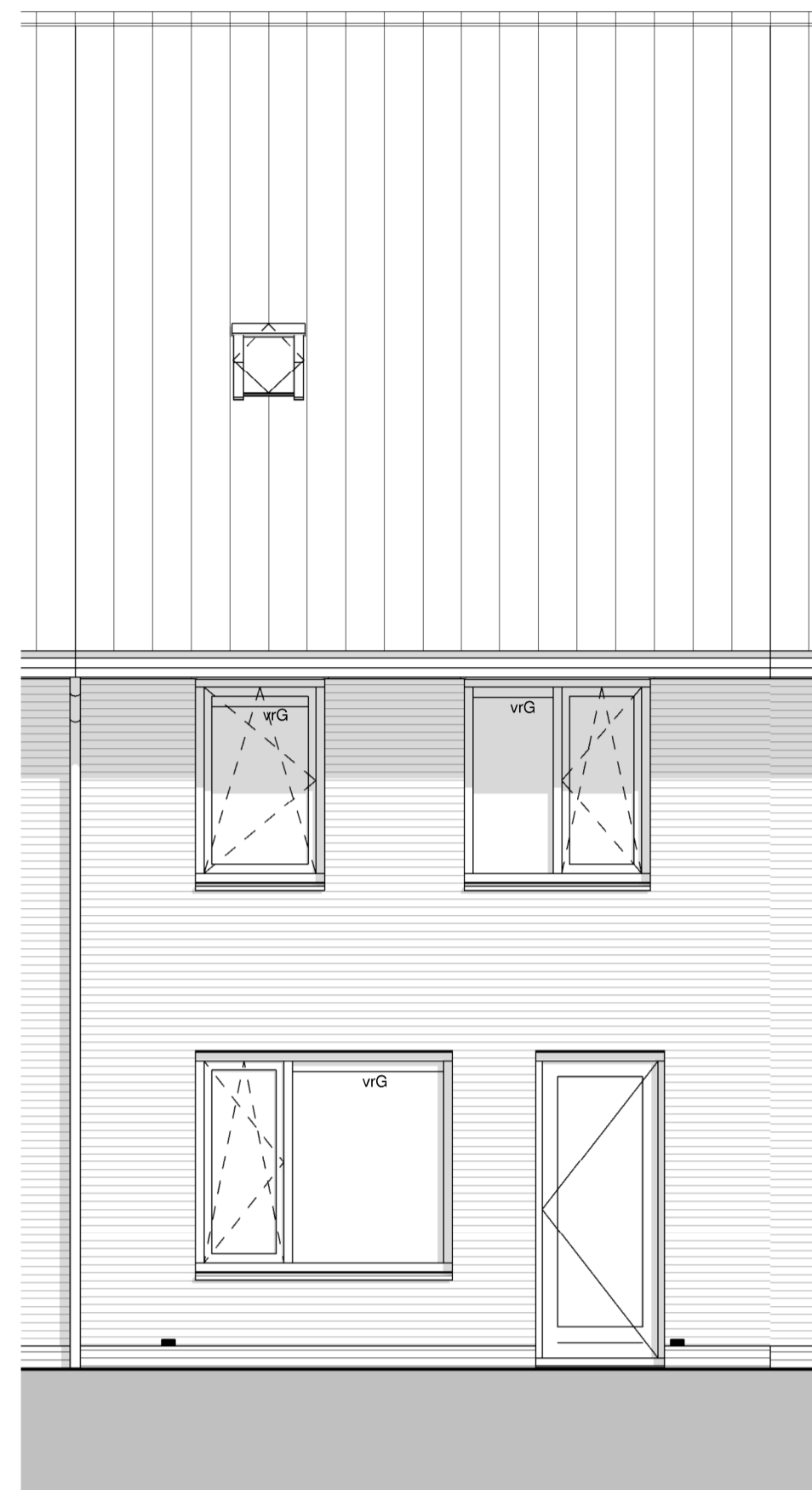
Achtergevel
