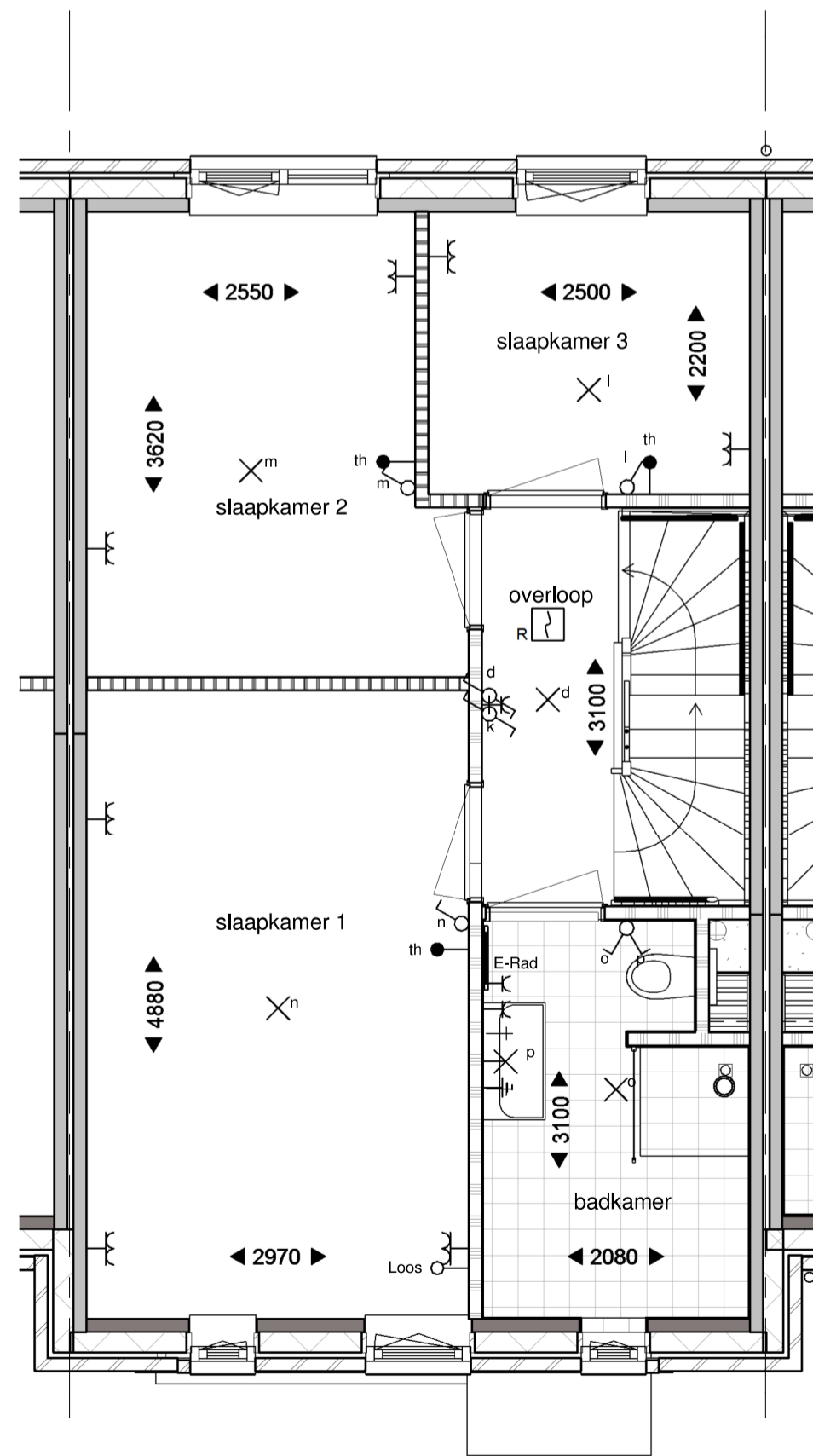
Eerste verdieping
