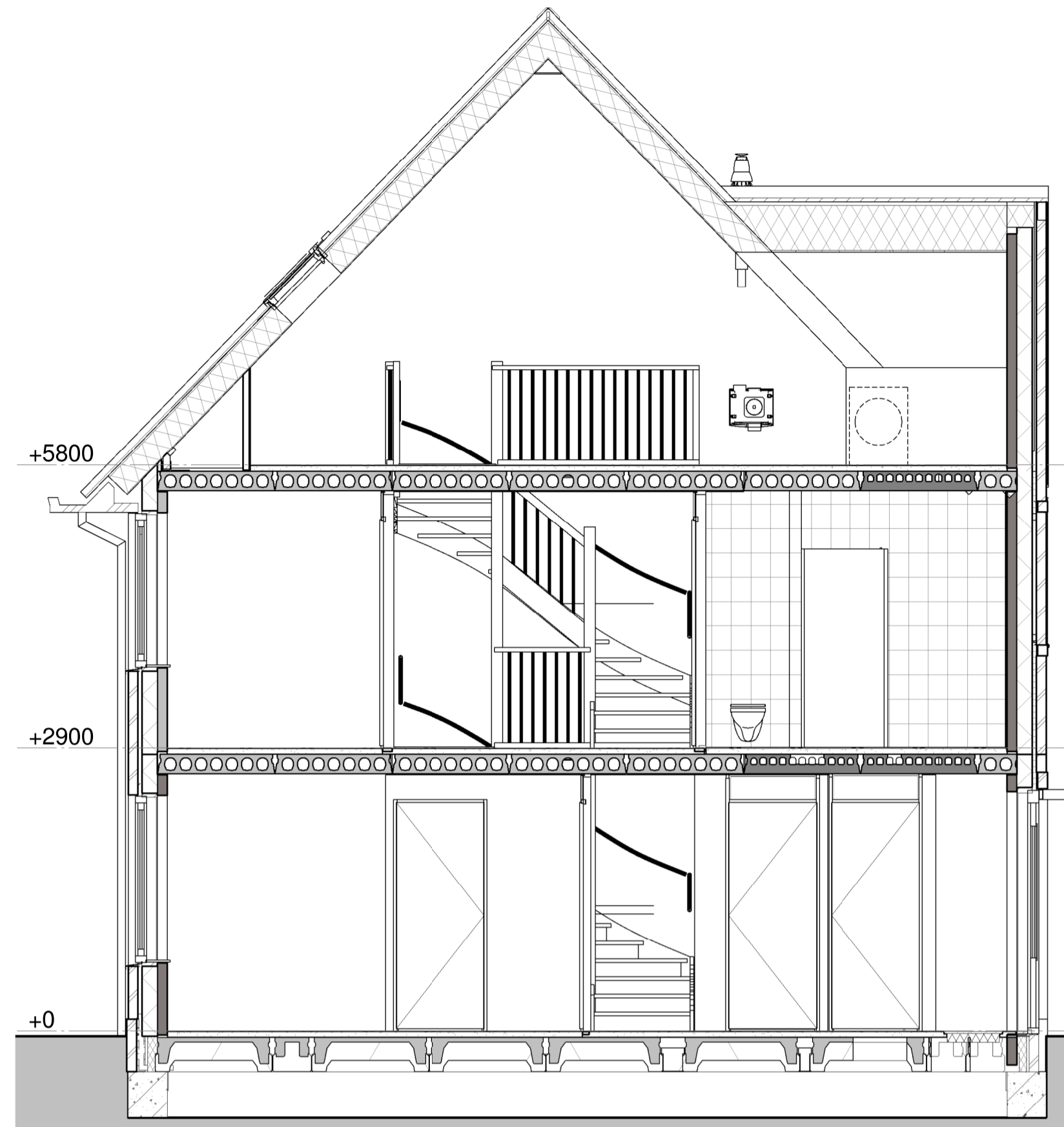
Doorsnede
