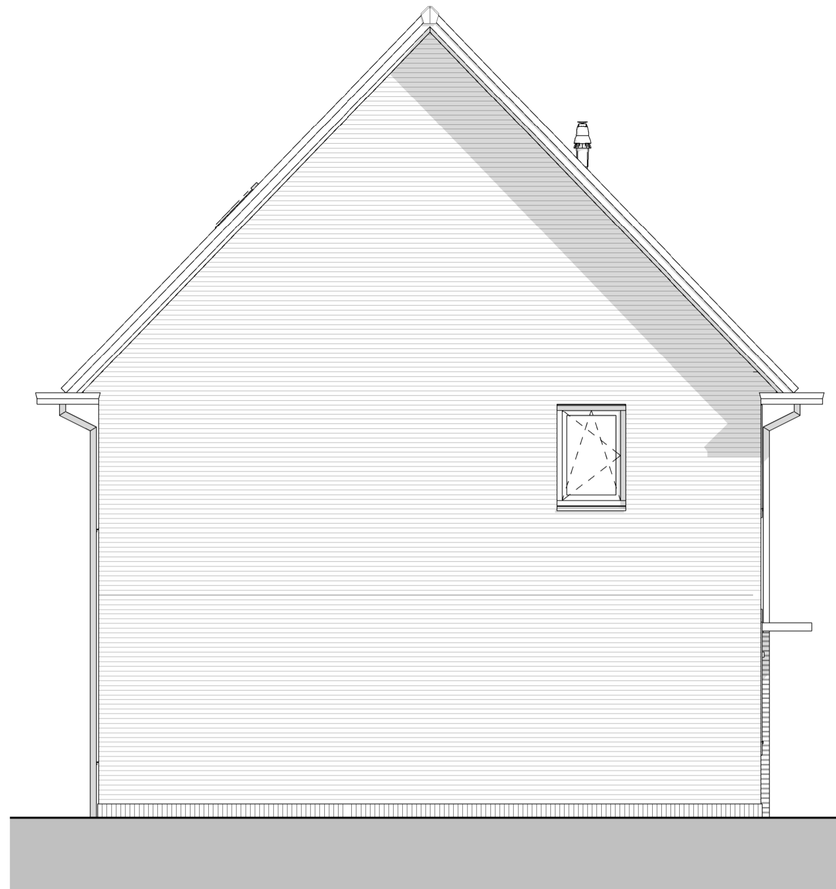
Linkergevel
