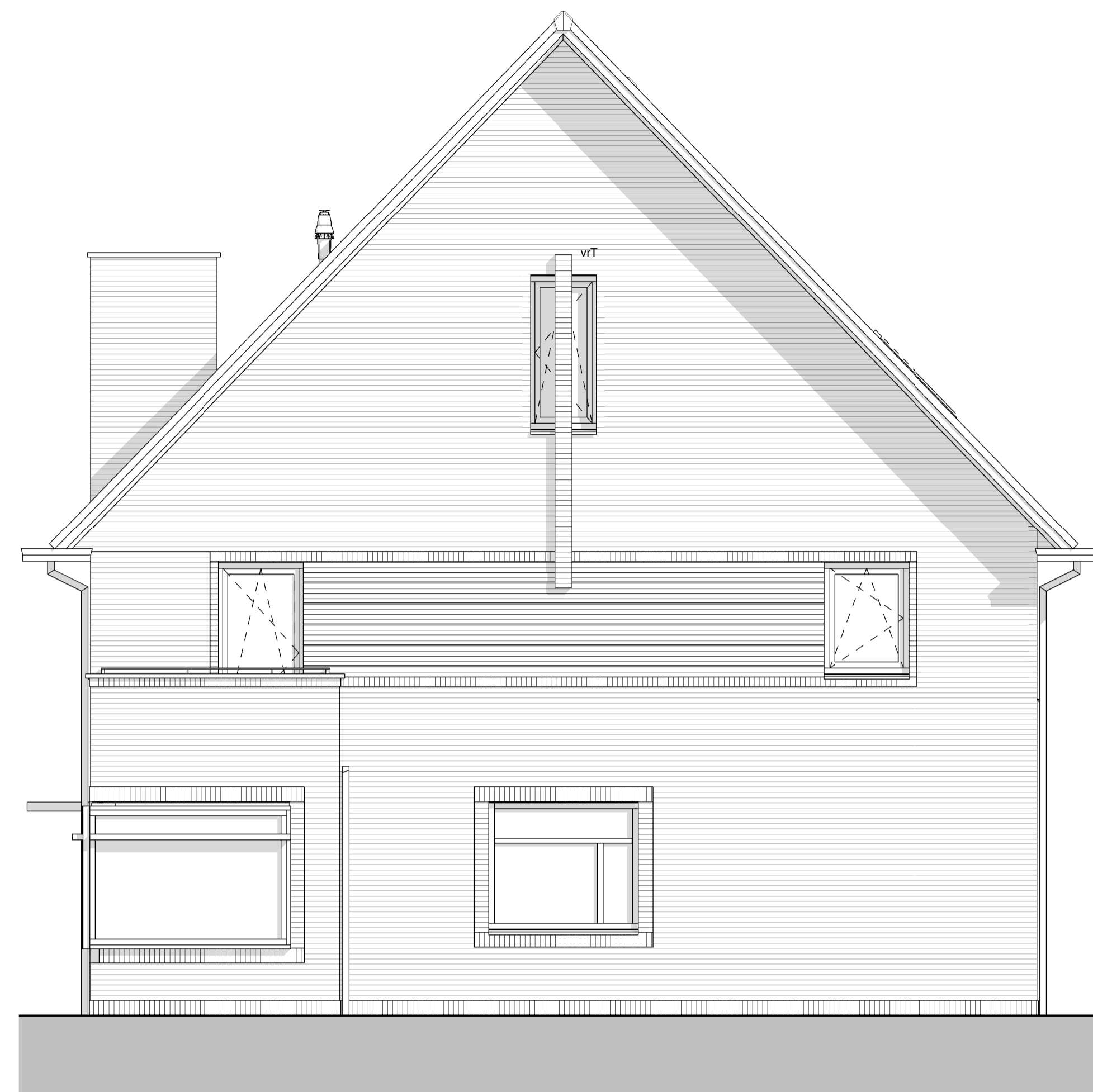
Rechtergevel
