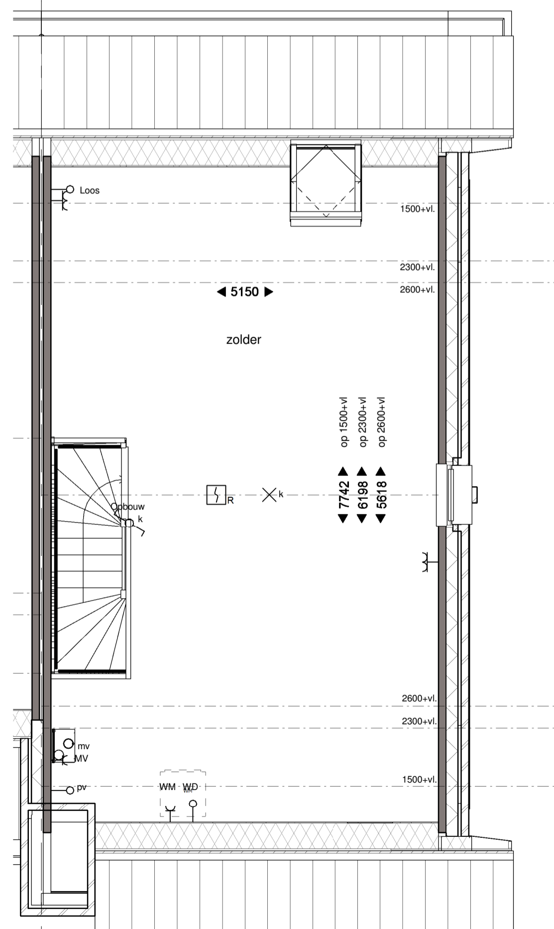
Tweede verdieping
