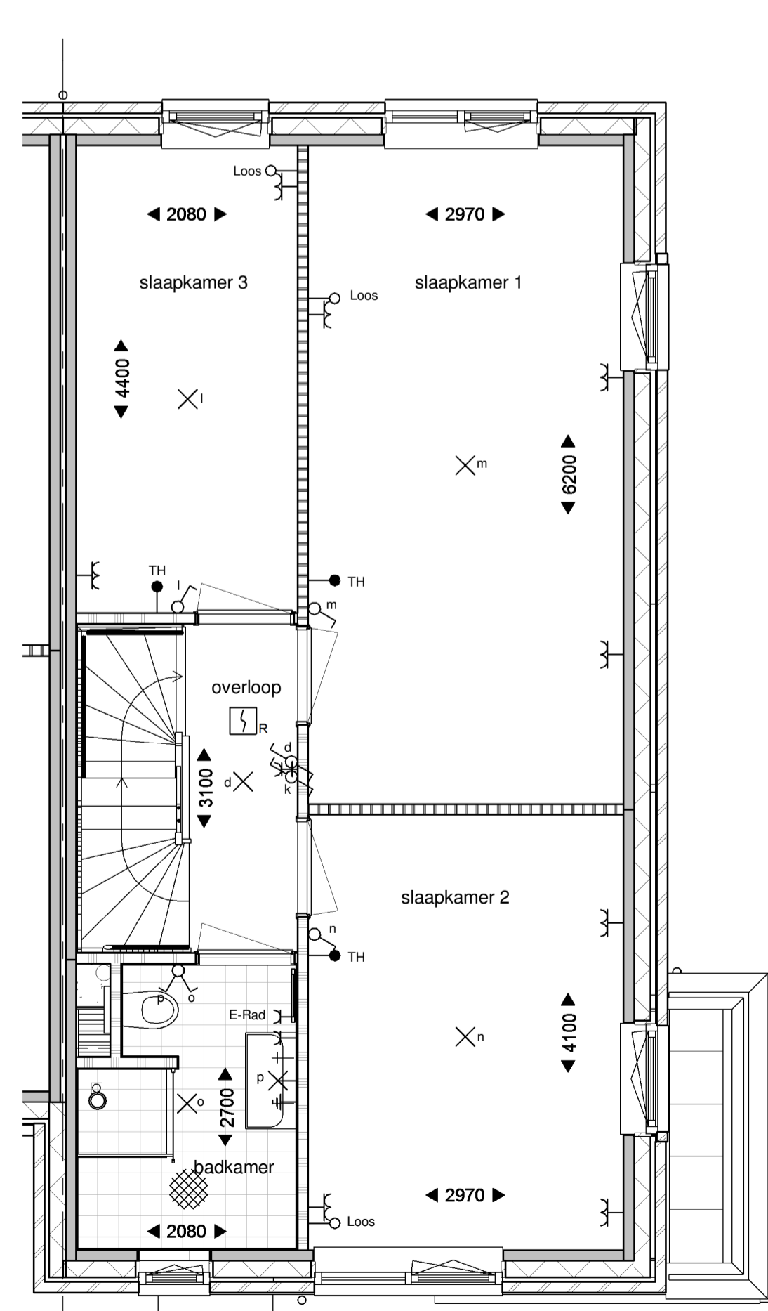
Eerste verdieping
