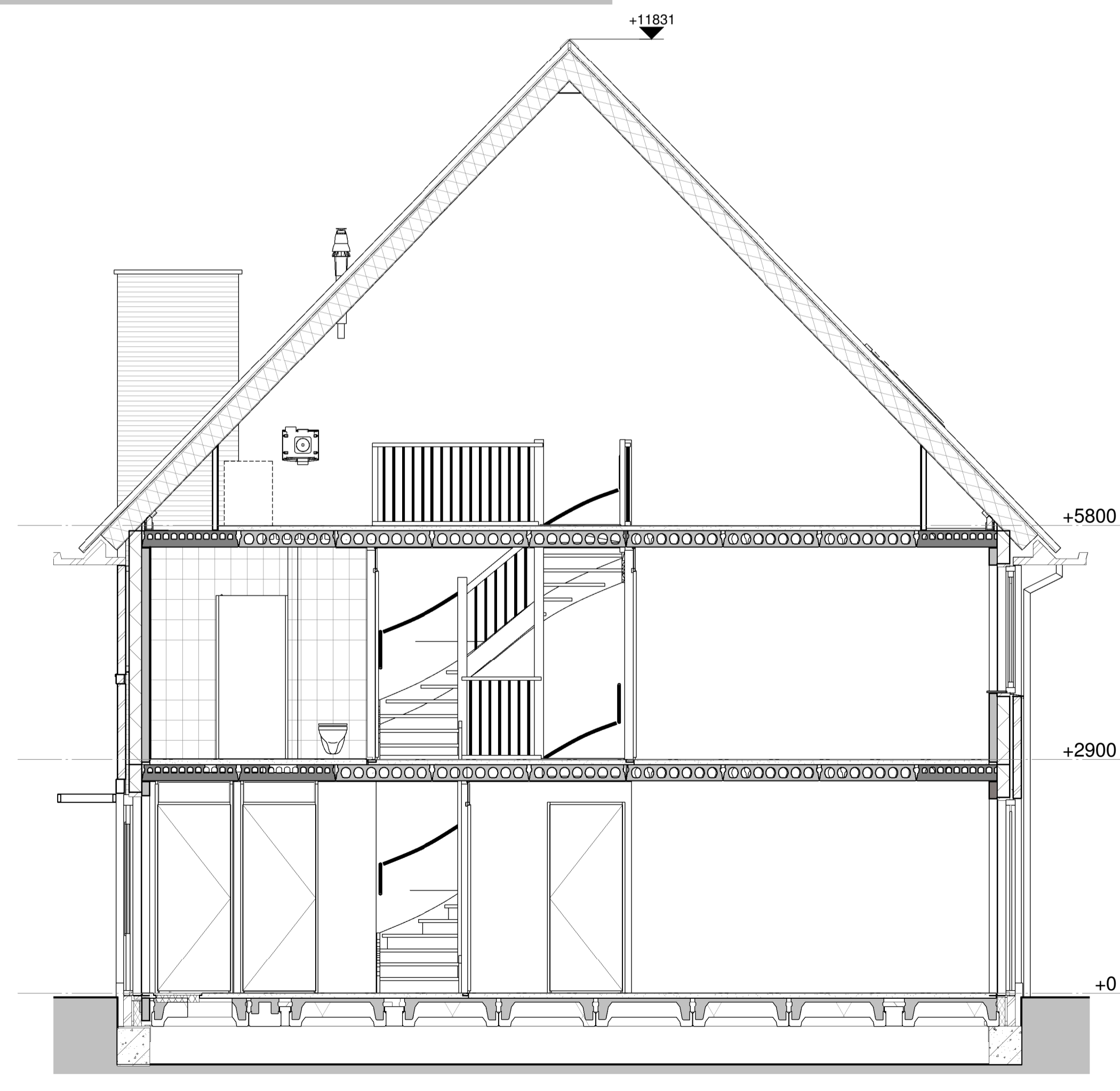
Doorsnede
