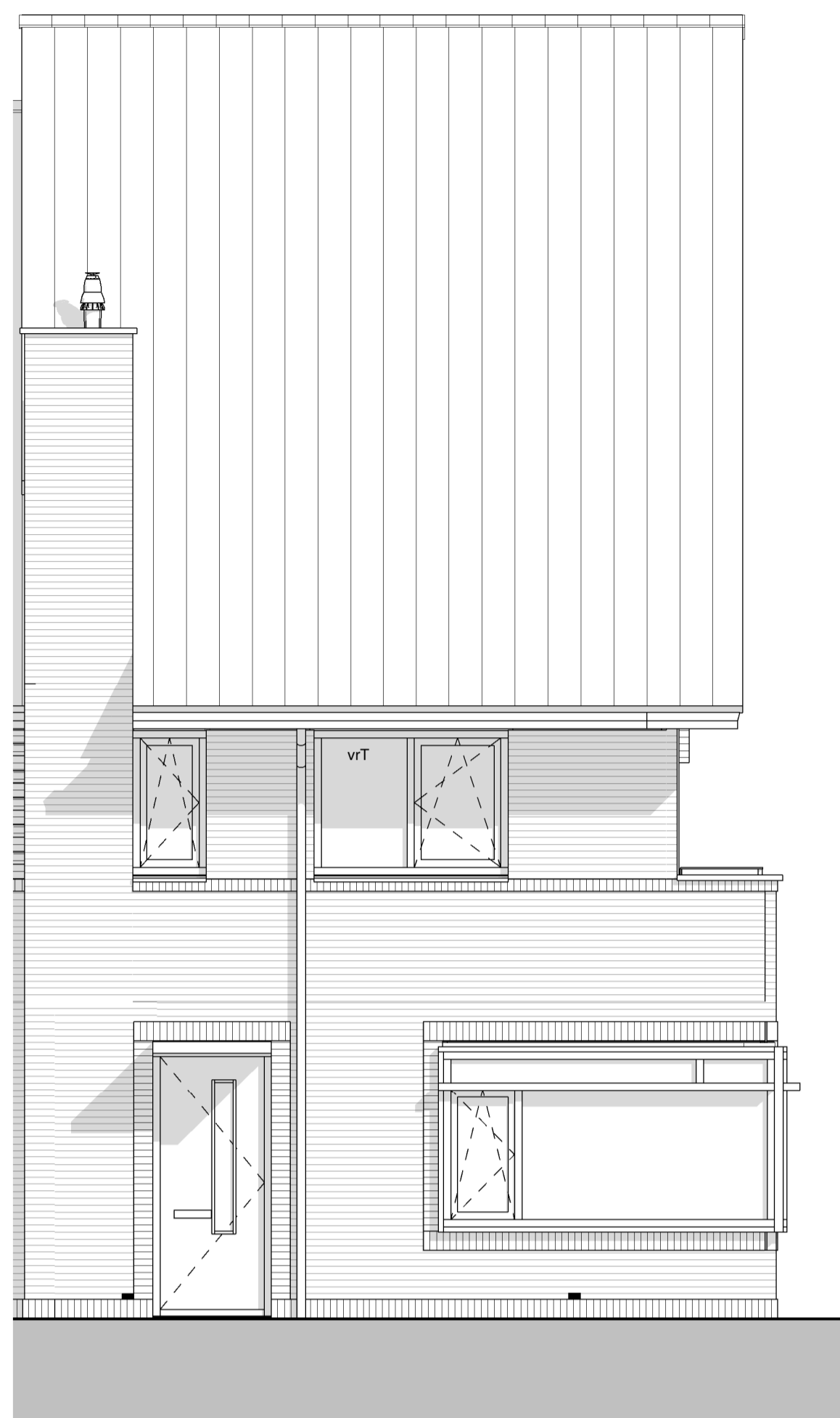
Voorgevel
