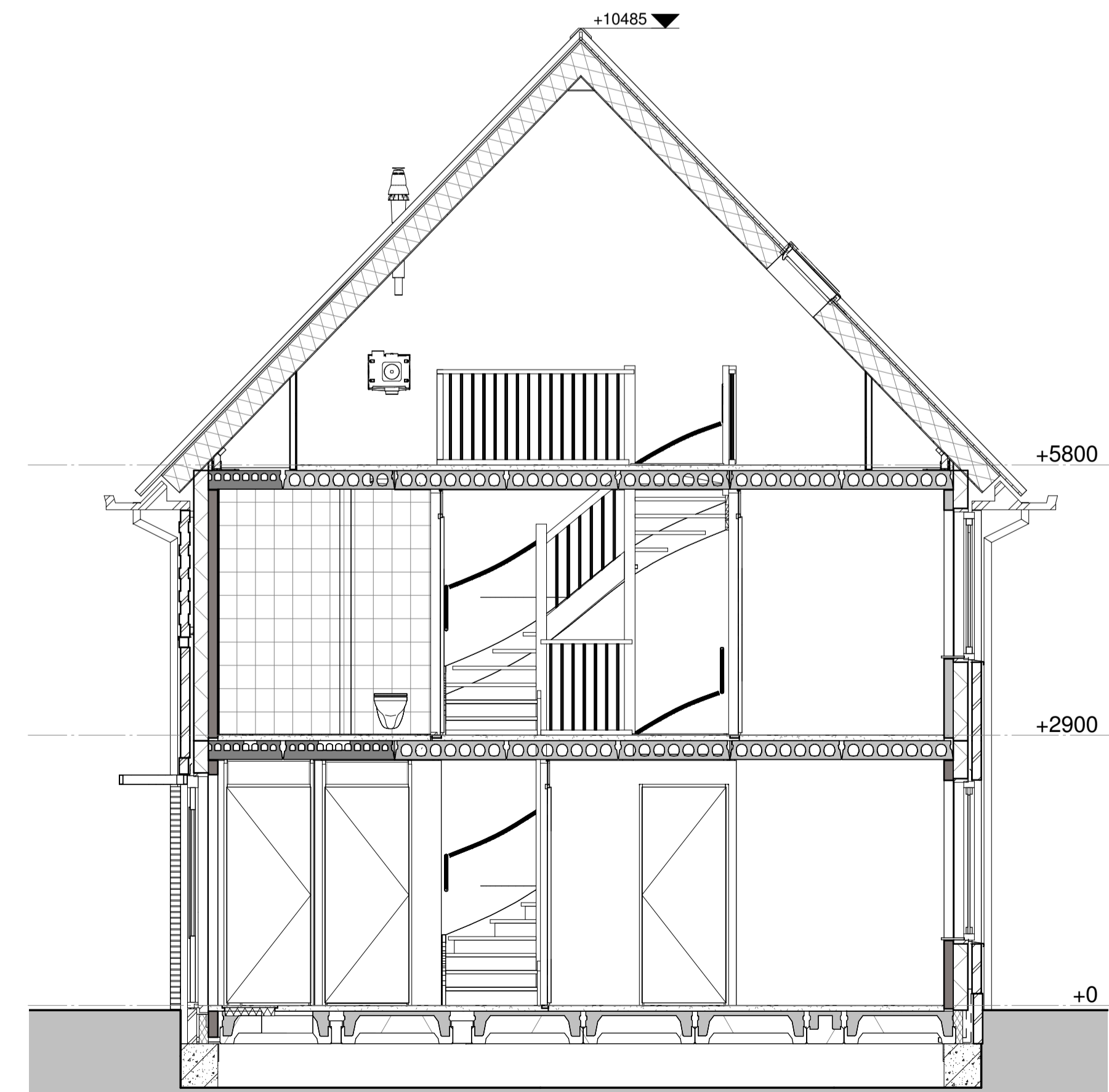
Doorsnede 21-B-B
