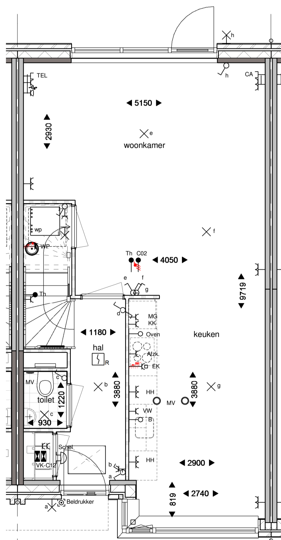
Begane grond
