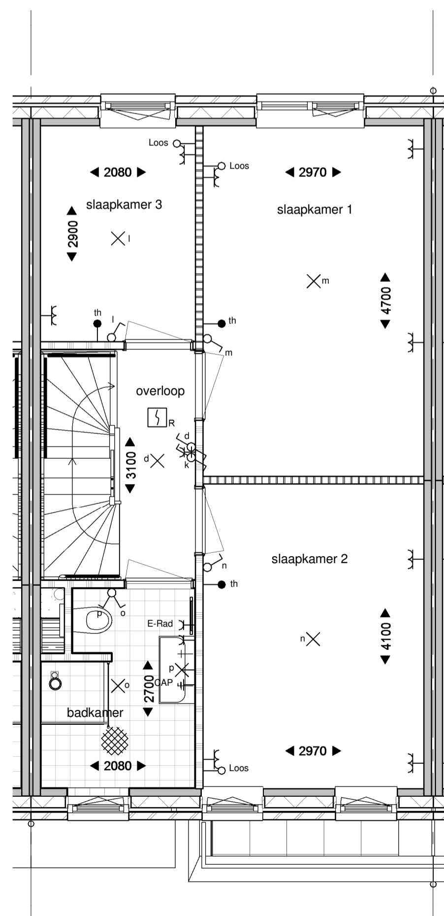
Eerste verdieping
