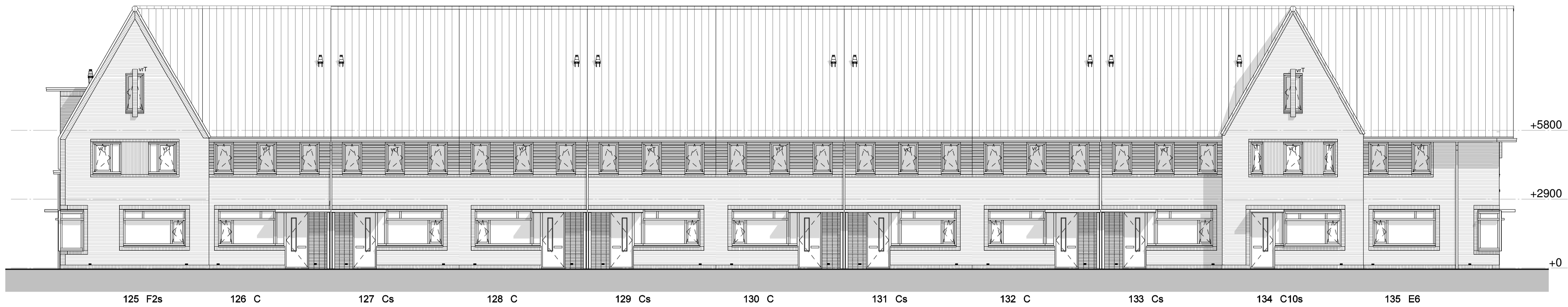
Voorgevel
