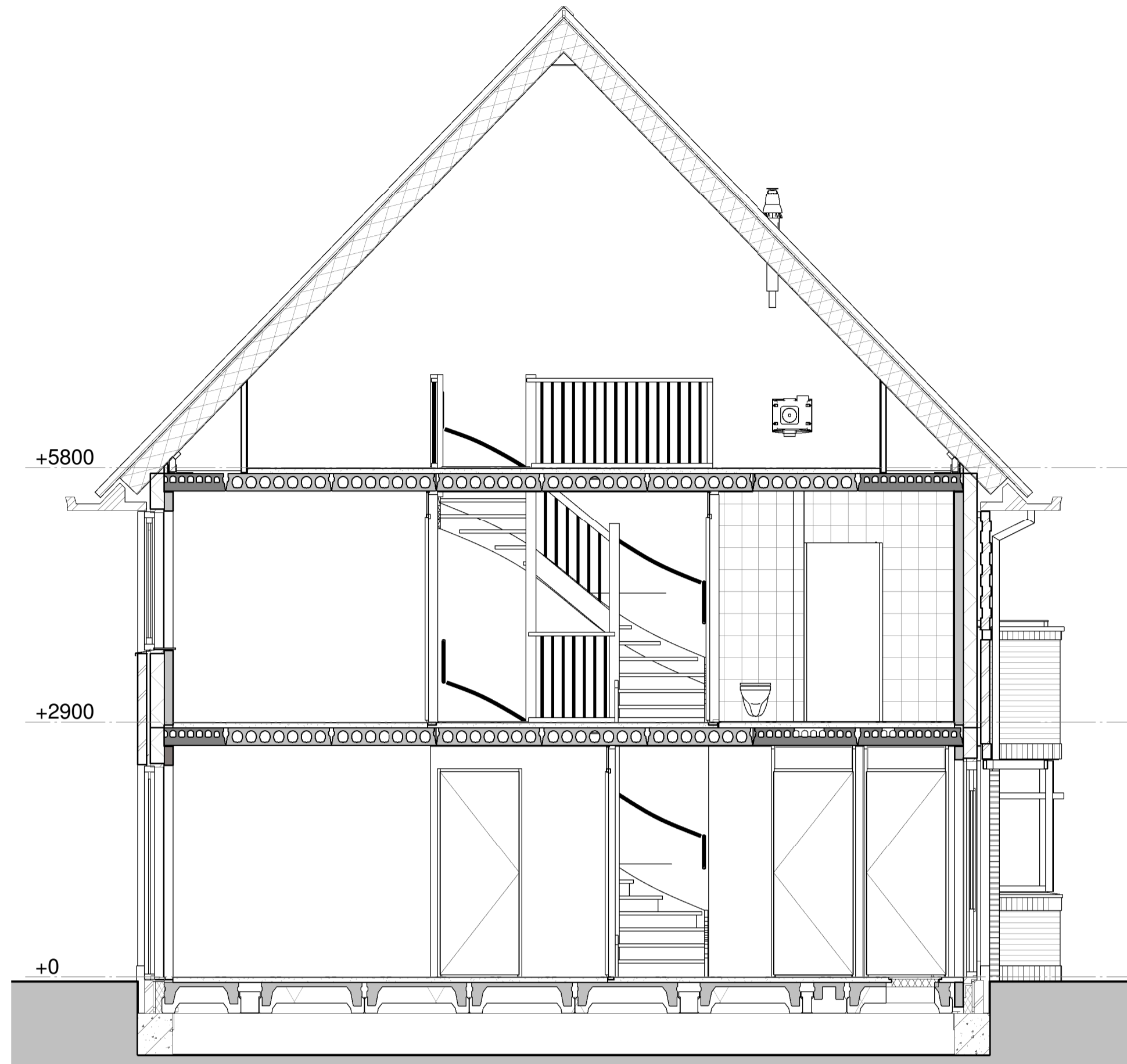
Doorsnede
