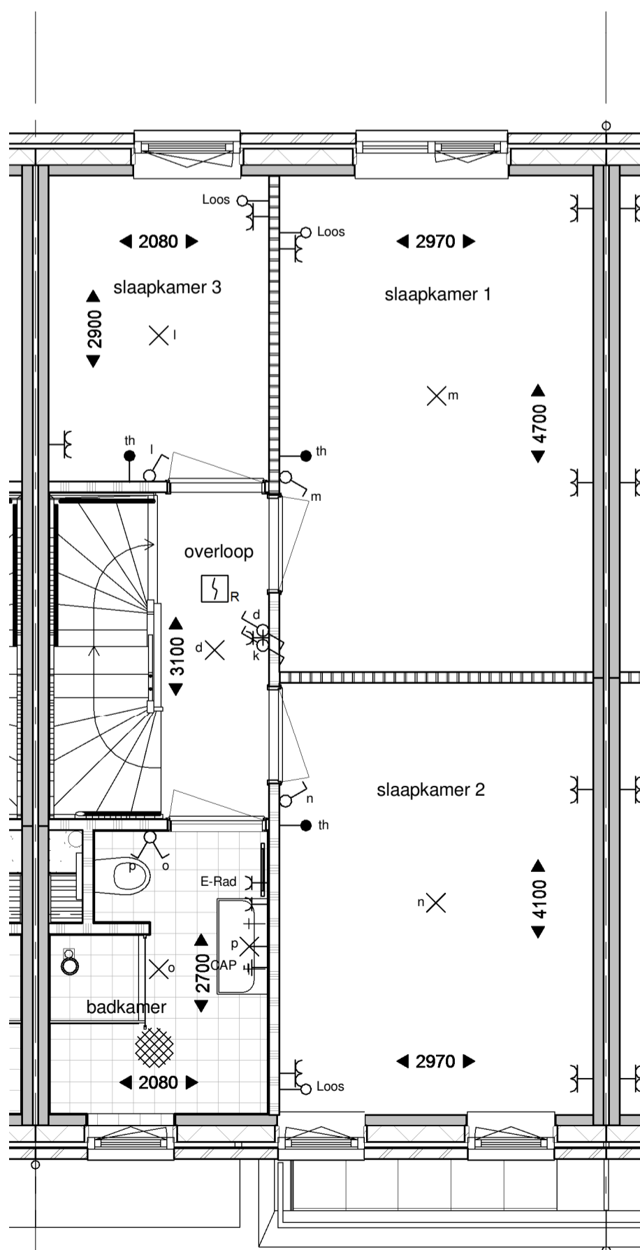
Eerste verdieping
